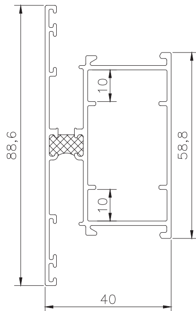
8304 HOJA PUERTA QT Peso : 1.253 Kg/M Espesor : 1.4 mm
