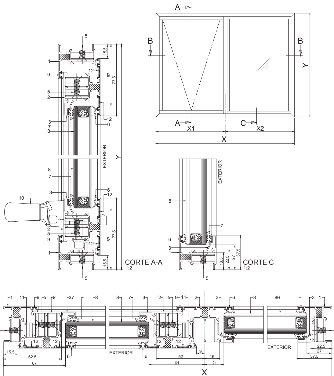
CORTE B-B 1:2
