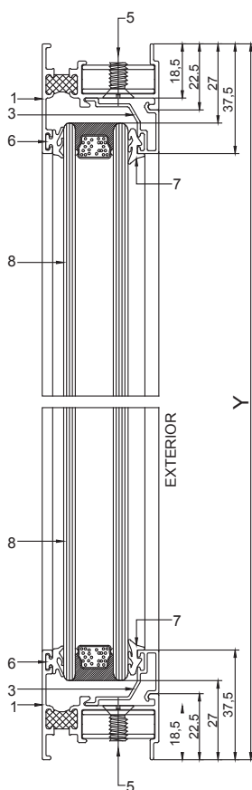
CORTE A-A 1:2
