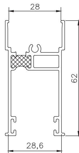
8904 ZOCALO/CABEZAL QT Peso : 0.903 Kg/M Espesor : 1.4 mm
