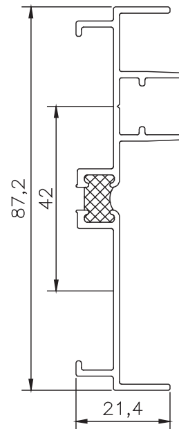
8903 JAMBA QT Peso : 0.800 Kg/M Espesor : 1.4 mm
